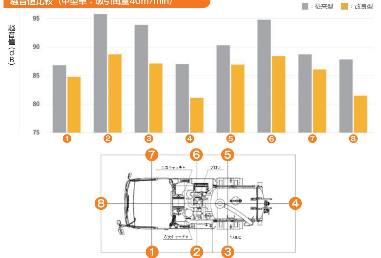
騒音値比較 (中型車：吸引風量40m 3 /min)
