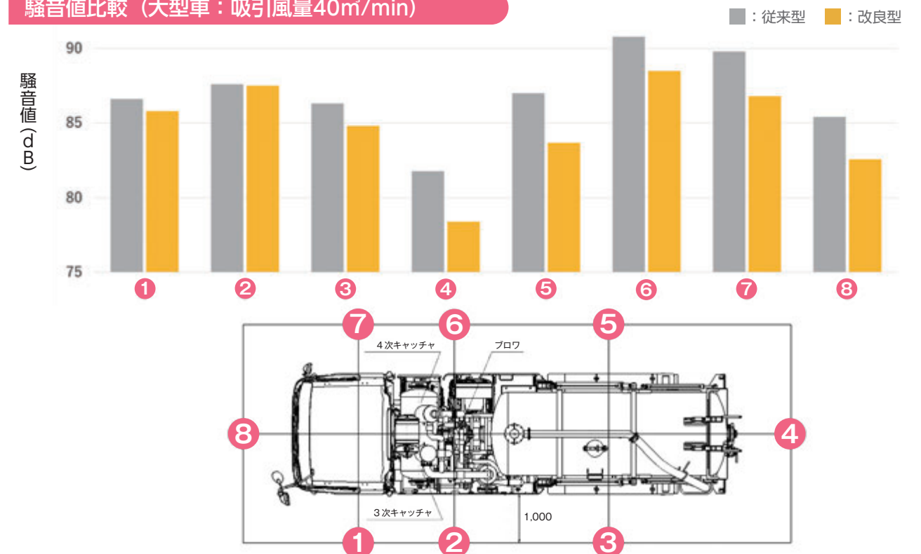
騒音値比較 (大型車：吸引風量40m 3 /min)
