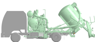
4トン 中型吸引車 SM-04BVP 風量：40m³/min
