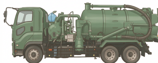
大型吸引車 SM-13CVP(風量40m 3 /min)
