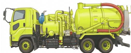
大型吸引車 SQ-13BVP(風量70m 3 /min)
