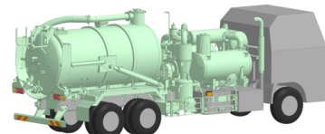
22トン 大型吸引車 SQ-13BVP 風量：70m³/min
