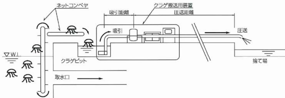
設置例
