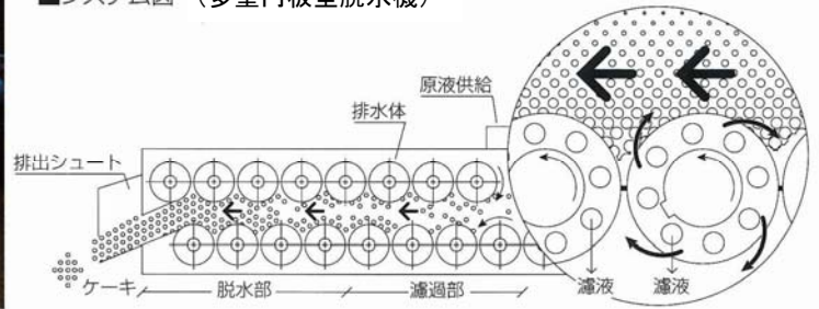
■システム図（多重円板型脱水機）
