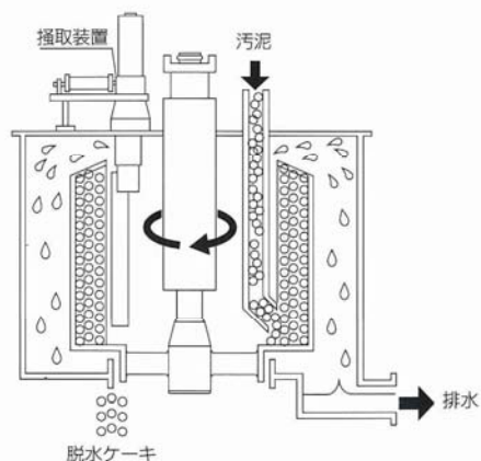
■システム図
