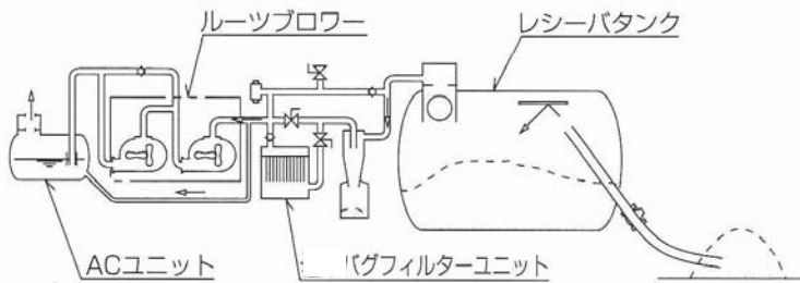
■システム図 (パワープロベスター・SQ-13DVFP)
