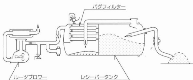
■システム図（乾式ルーツブロワー搭載車）
